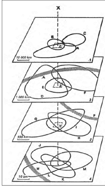
Şekil 4. Lacoste’un diatopik yönteminin şematize edilmesi (Lacoste, 2014).
